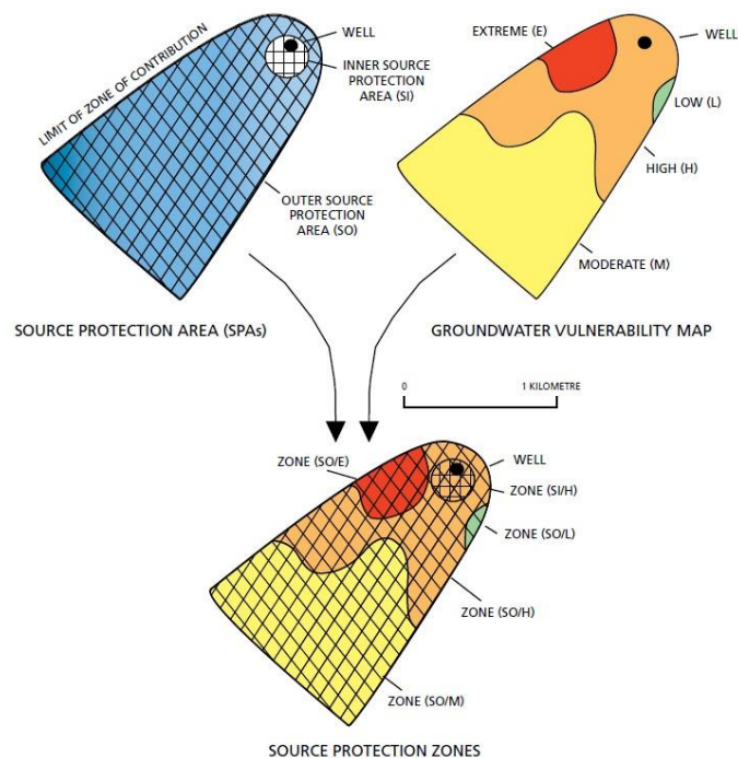
Slika 7. Definiiranje zaštitnih zona izvorišta (DELG/EPA/GSI, 1999)
