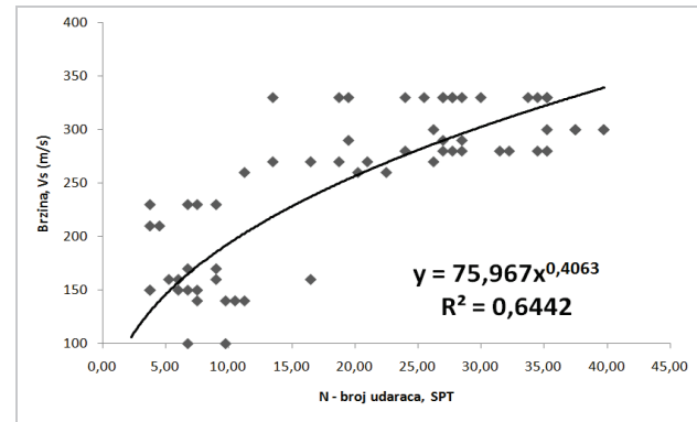
Slika 21. Korelacija v_s = f(N_{60SPT}) za istraživane krupnozrne šljunke
