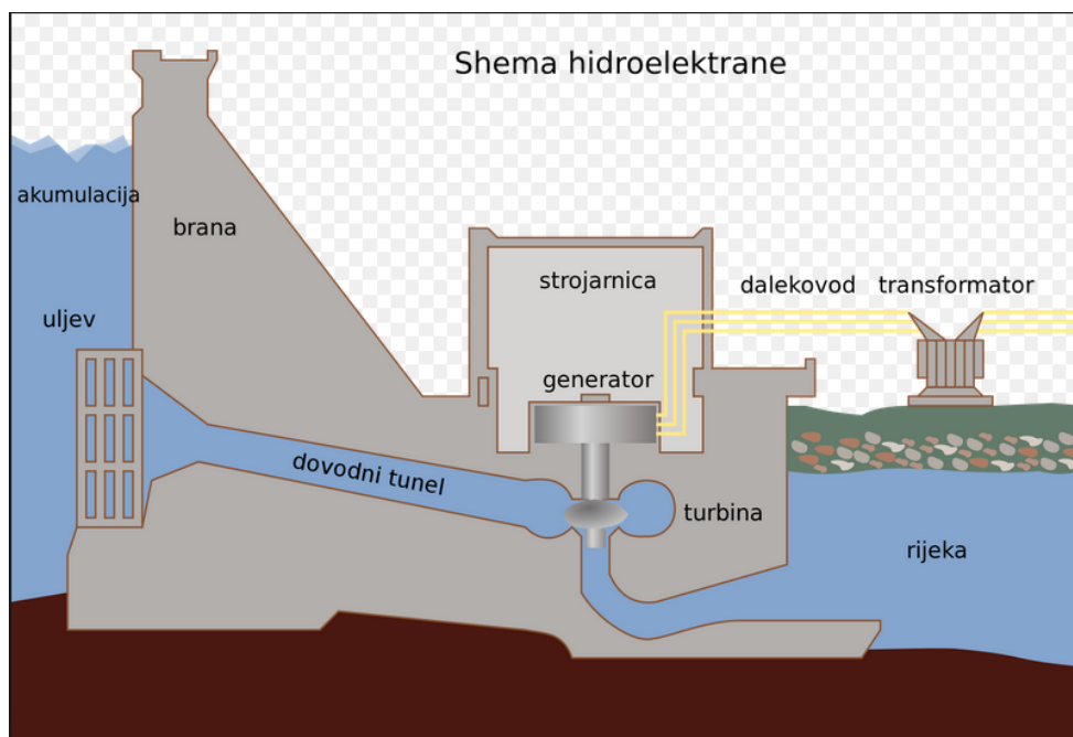
Slika 14. Shema hidroelektrane [10]
