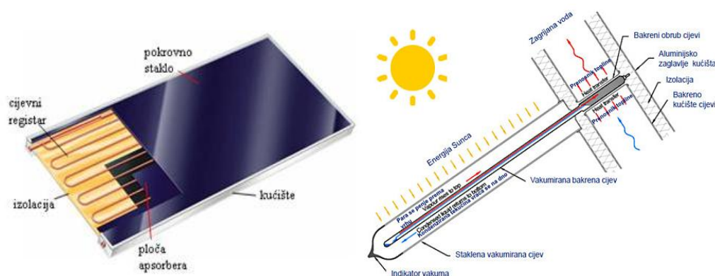
Slika 5. Pločasti i vakuumski kolektor [4]
