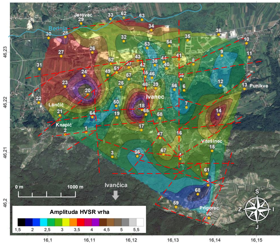
Slika 26. Karta HVSr amplituda sedimenata na području grada Ivanca: a) konture amplituda projicirane na satelitsku snimku područja, b) konture amplituda s označenim rasjedima s osnovne geološke karte. Žutim krugovima je označeno 68 lokacija HVSr mjerenja.
