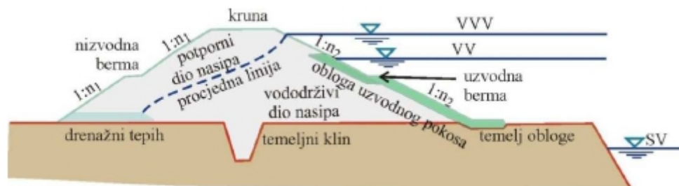
Slika 2. Hidrotehnički nasip [3]
