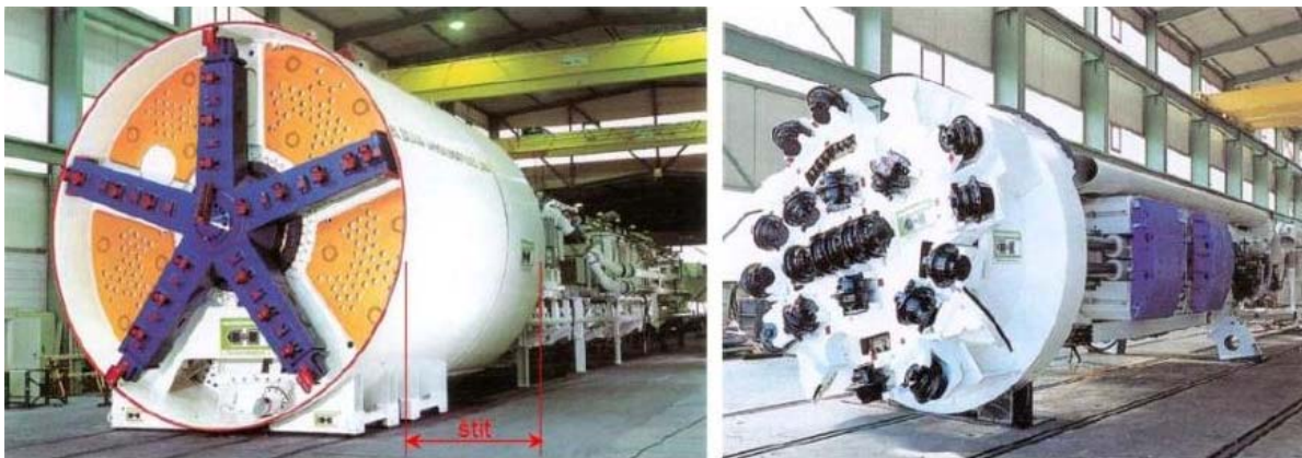
Slika 7.2 Stroj sa i bez štita
