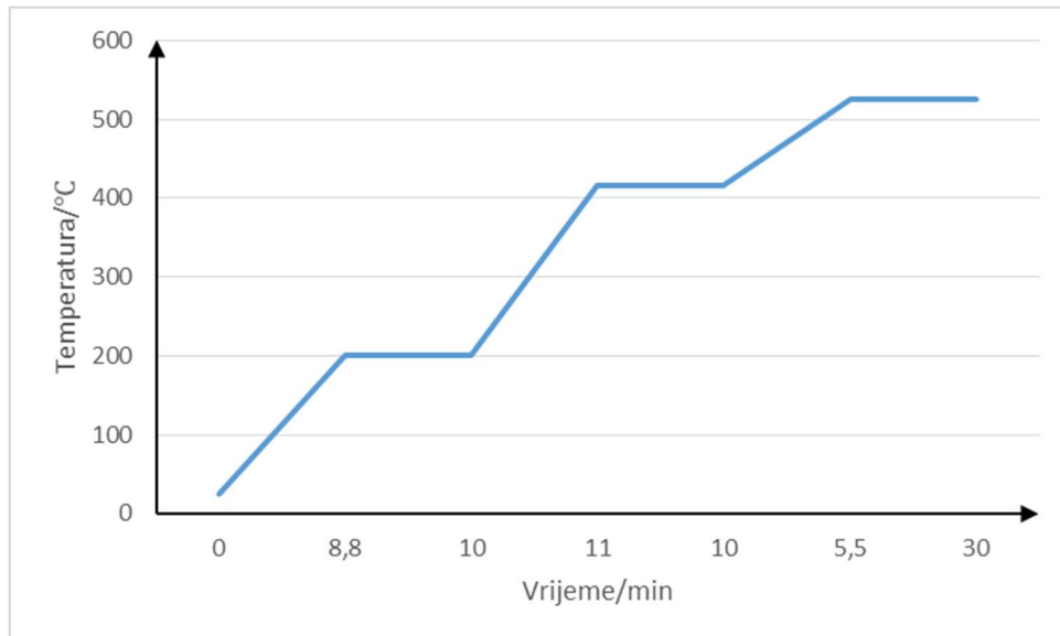
Slika 10: Temperaturni dijagram koji je određen za provođenje vakuumске pirolize
