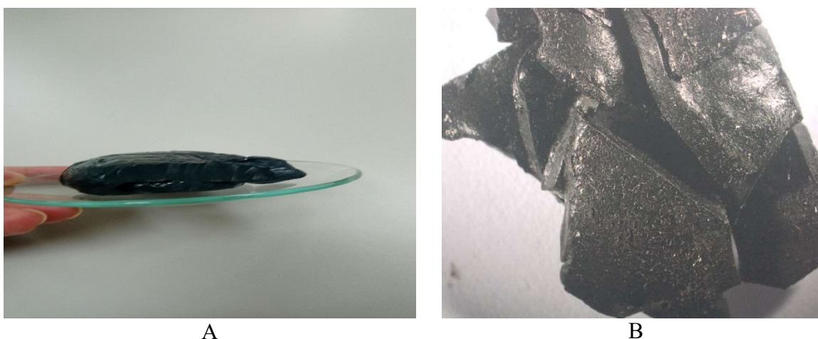
Slika 12: Prikaz uzorka mulja prije (A) i nakon (B) vakuumske pirolize
