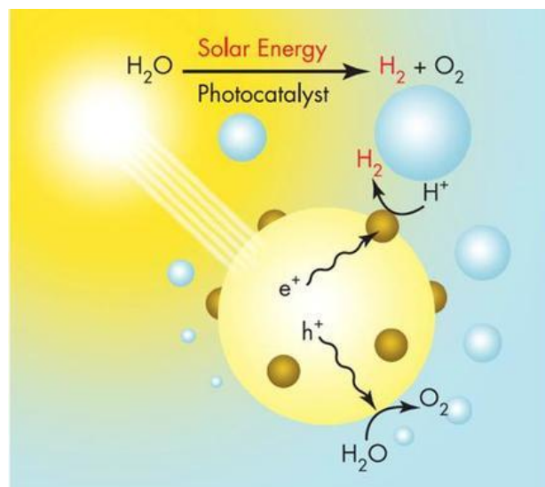
Slika 17. Solarna fotokataliza [20]
