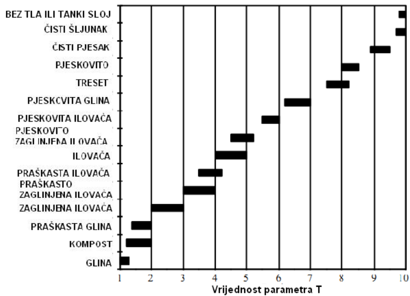
Slika 9. Dijagram određivanja parametra T (prema: Civita & De Maio, 2000 )
