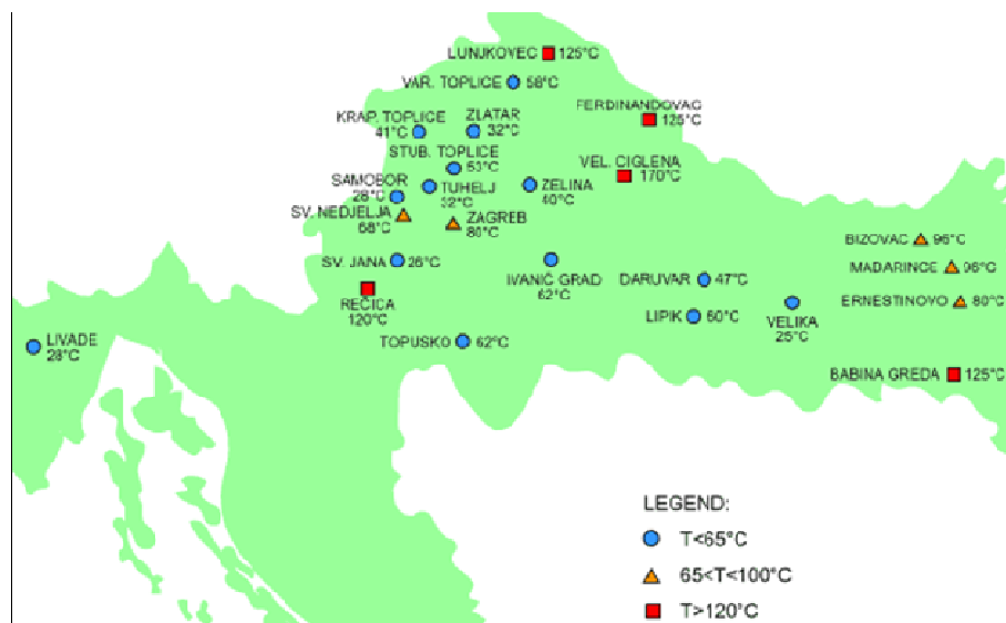
Slika 3. Temperature geotermalnih ležišta panonskog dijela RH. [6]
