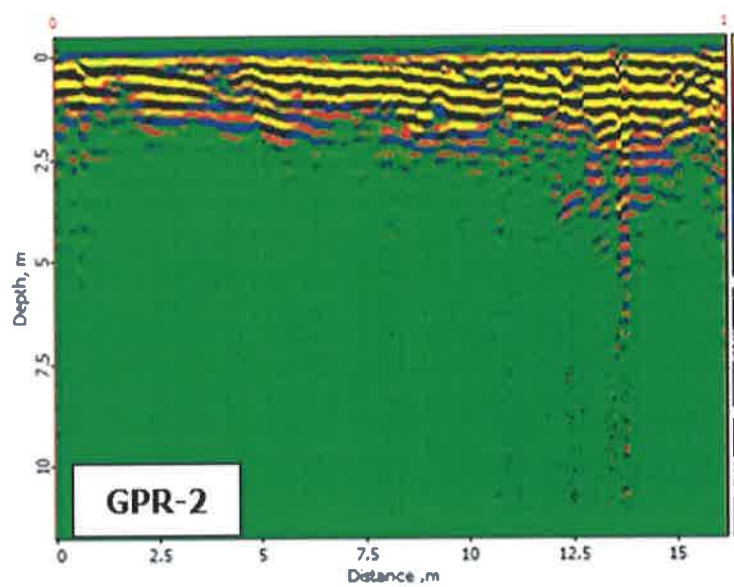
Slika 25. Rezultat georadarskog profiliranja profila GPR-2 (Strelec et al., 2013)
