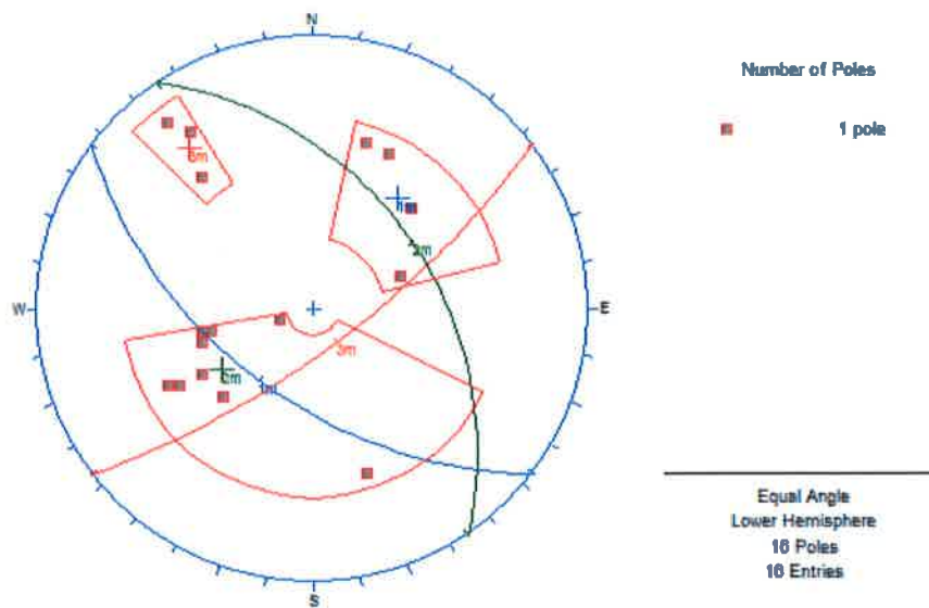
Slika 16. Kumulativni dijagram trasa ravnina pukotina i rasjeda mjeren u zoni Kule Minčeta jedinice, slojni diskontinuiteti - zeleno, osna ravnina – plavo, okomito na os „b“ - crveno.
