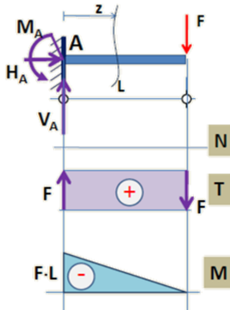
Slika 25. MNT dijagram
