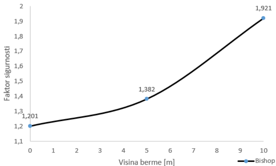
Slika 24. Utjecaj promjene visine berme na faktor sigurnosti [11]
