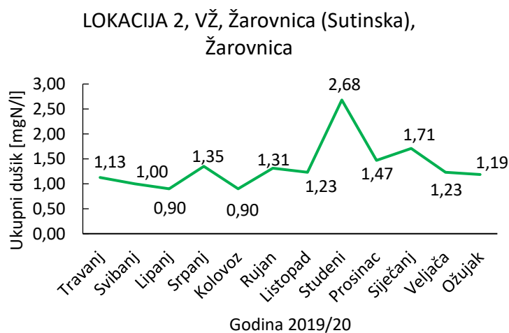
Slika 13. Grafički prikaz vrijednosti ukupnog dušika za lokaciju 2 Varaždinske županije za razdoblje od travnja 2019. do ožujka 2020. godine
