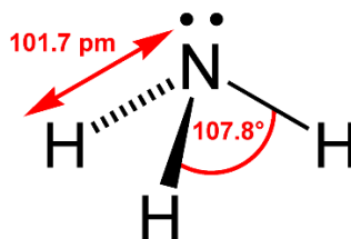
Slika 2. Struktura amonijaka
