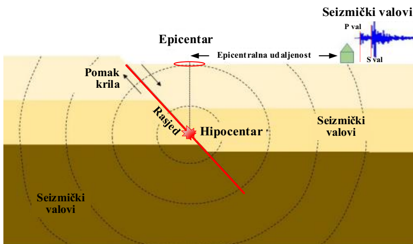
Slika 4. Opis nastanka potresa pri pomaku dva bloka duž rasjeda (Kentucky Geological Survey, 2018)
