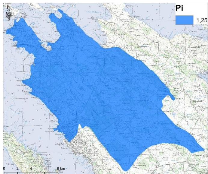
Slika 16. Podfaktor P_i određen za sliv Bokanjac – Poličnik
