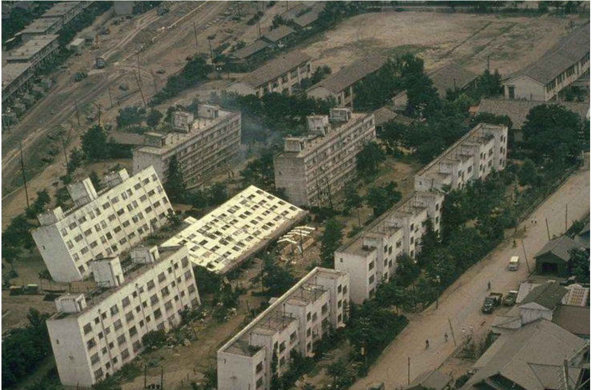
Slika 7 Prevrtnje građevina uzrokovano likvefakcijom tla (Geotech, 2019.)
