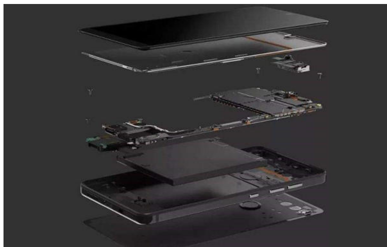
Slika 5: Kućište mobitela [26]
