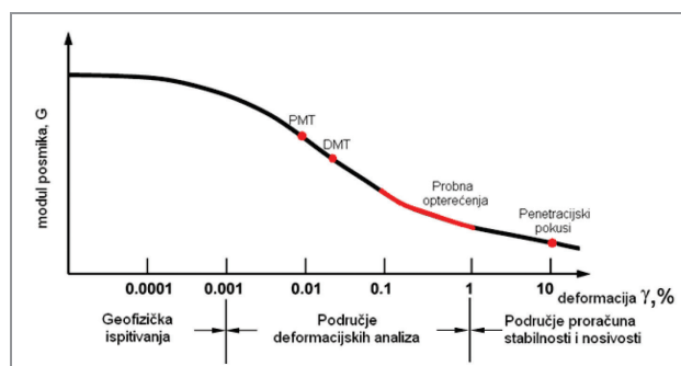
Slika 2. Raspodjela krutosti tla u ovisnosti o veličini deformacija i metodi ispitivanja (Luna, R., Jaji, H., 2000.)
