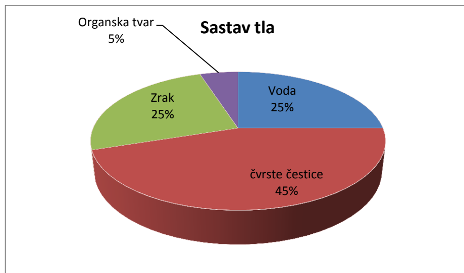
Slika 2.Sastav tla
