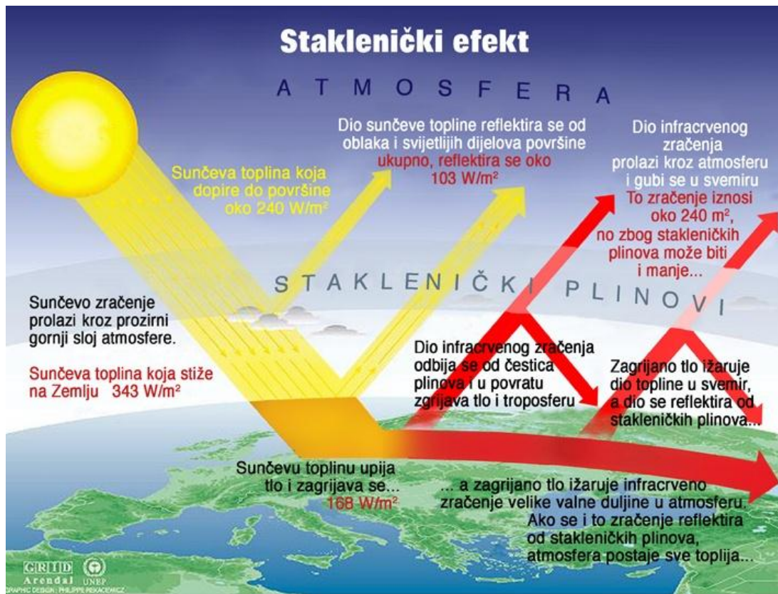
Slika 1. Efekt staklenika
