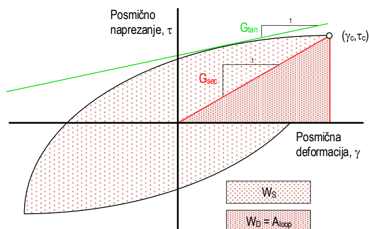
Slika 7. Ekvivalentni linearni model, hysteretička krivulja (histereza) odnosa naprezanja i deformacija.
