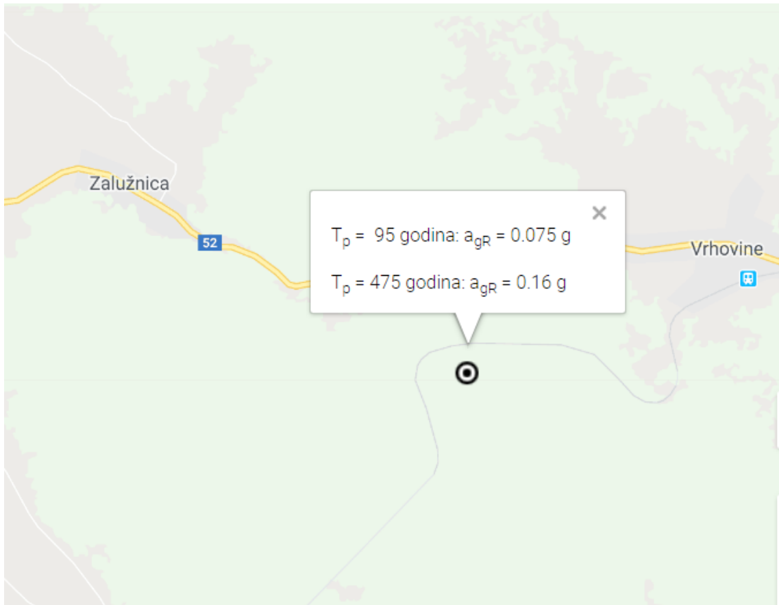
Slika 9. Isječak karte Republike Hrvatske sa srednjim vrijednostima akceleracije
