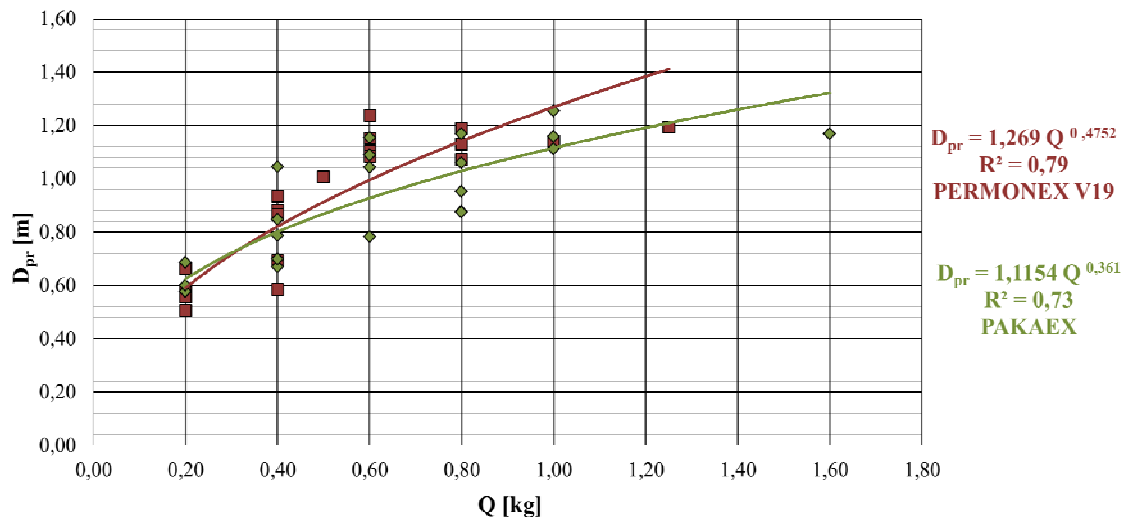
Slika 10.3 Dijagram ovisnosti promjera proširenja D_{pr} [m] o masi eksplozivnog punjenja Q [kg], Permonex V19 i Pakaex, za 2014., 2015. i 2016. godinu.
