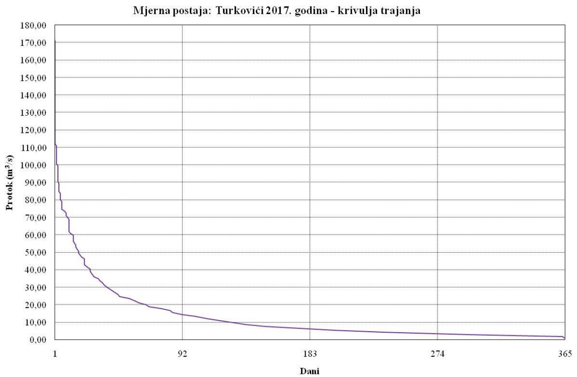
Slika P3-9. Grafički prikaz krivulje trajanja protoka na lokaciji Turkovići za 2017. godinu
