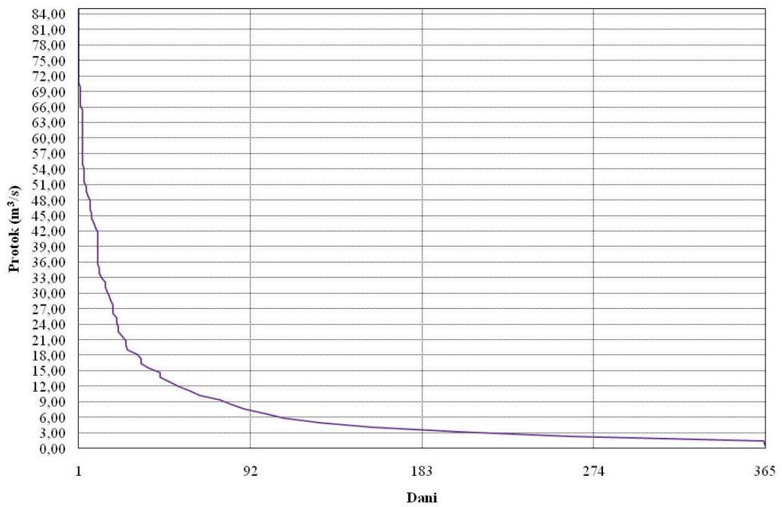
Mjerna postaja: Luke, 2017. godina - krivulja trajanja
