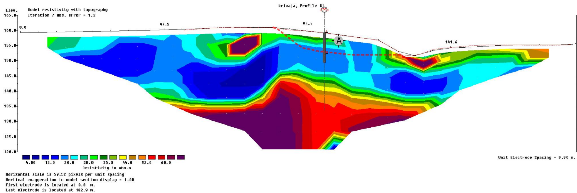
Slika 31. Model otpornosti u profilu elektricne tomografije ERT-1 Krivaja
