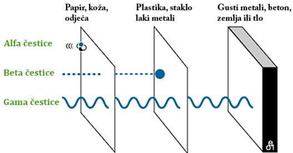
Slika 1. Prodornost zračenja [5]
