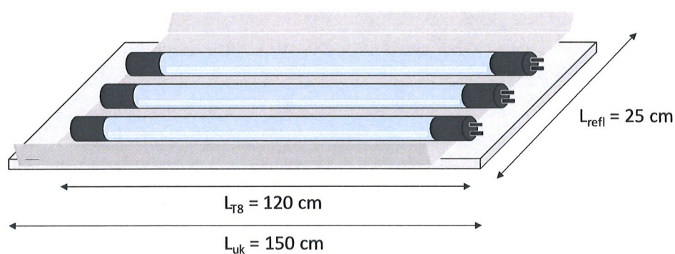
Slika 6. Postav izvora zračenja s dimenzijama
