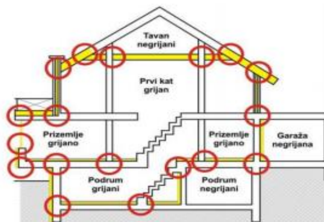
Slika 8. Tipična mjesta pojave toplinskih mostova u konstrukciji [15]
