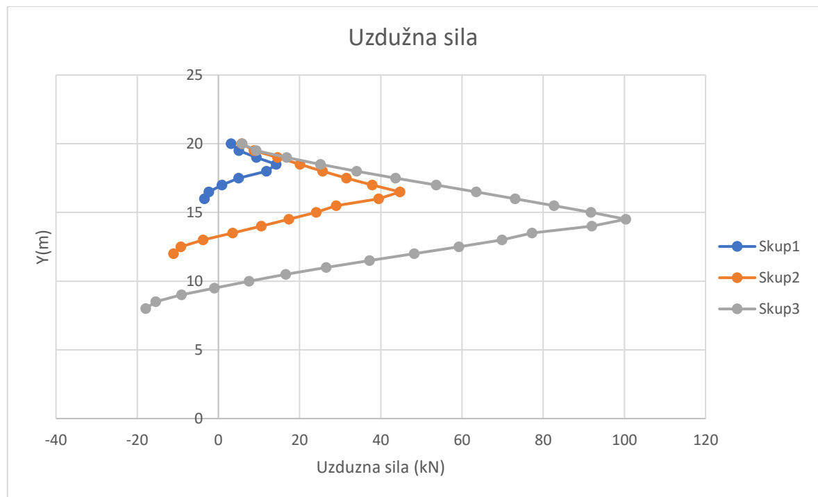
Dijagram 5. Uzdužna sila
