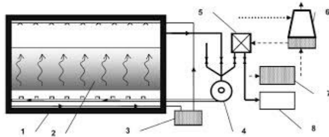
Slika 5. Shematski prikaz zatvorenog spremnika za biosušenje temeljeno na Herhof-om sustavu [10]
