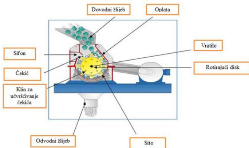
Slika 7: Mlin čekičar s osnovnim dijelovima
