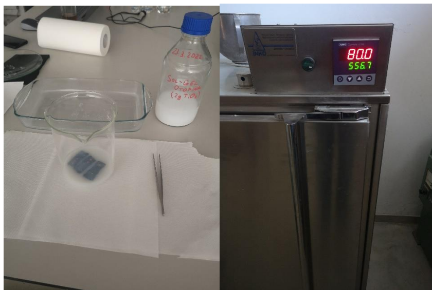
Slika 9. Umakanje gumenih podloga u pripremljenoj sol-gel otopini (lijevo) i prikaz sušionika zagrijanog na potrebnu temperaturu za sušenje gumenih podloga (desno)
