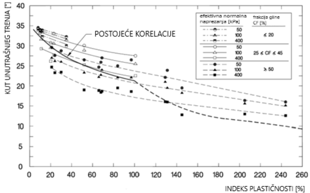
Slika 18 – korelacija I_p - \Phi za rekonstituirane normalno konsolidirane gline kao u zavisnosti frakcije gline CF i efektivnog normalnog naprezanja \sigma'_n [20]
