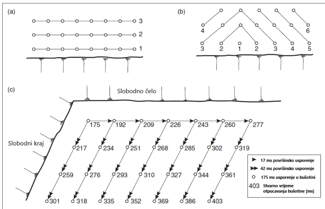
Slika 15. Redosljedni detonacije: (a) kvadratni redosljed detonacije "red po red"; (b) uglat "V" redosljed detonacije; (c) milisekundno otpucavanje minskih bušotina (preađeno prema [13])
