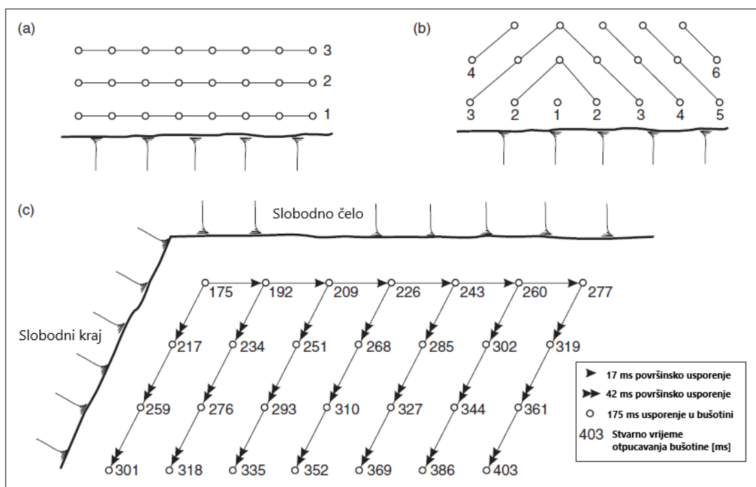
Slika 15. Redosljedi detonacije: (a) kvadratni redosljedi detonacije "red po red"; (b) uglat "V" redosljedi detonacije; (c) milisekundno otpucavanje minskih bušotina (preađeno prema [13])
