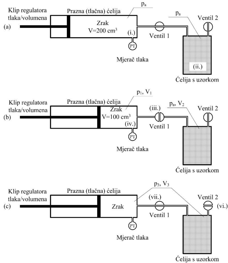
Slika 34. Shematski prikaz mjerenja modifikiranim plinskim piknometrom konstantnog volumena
