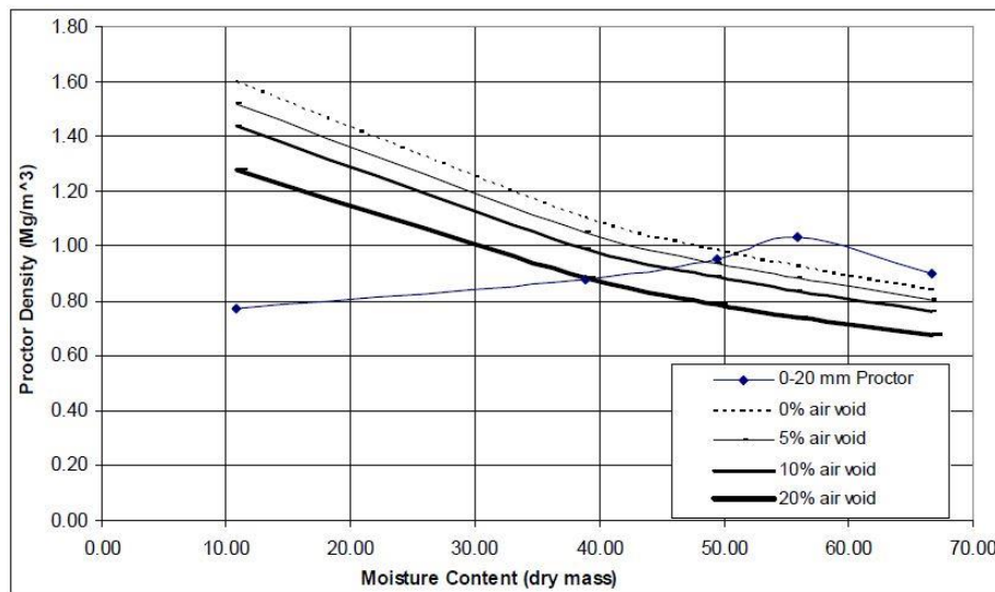
Slika 48. Krivulja zbijanja frakcije 0-20 mm (Sudarshana, 2011) (Prijevod: Os x – moisture content (dry mass) – udio vlage izražen preko suhe mase; Os y – proctor density ( \text{g/cm}^3 ) – suha gustoća ( \text{g/cm}^3 ))
