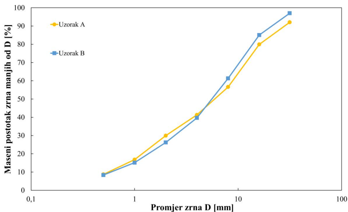
Slika 25. Granulometrijske krivulje uzoraka bioosušenog otpada
