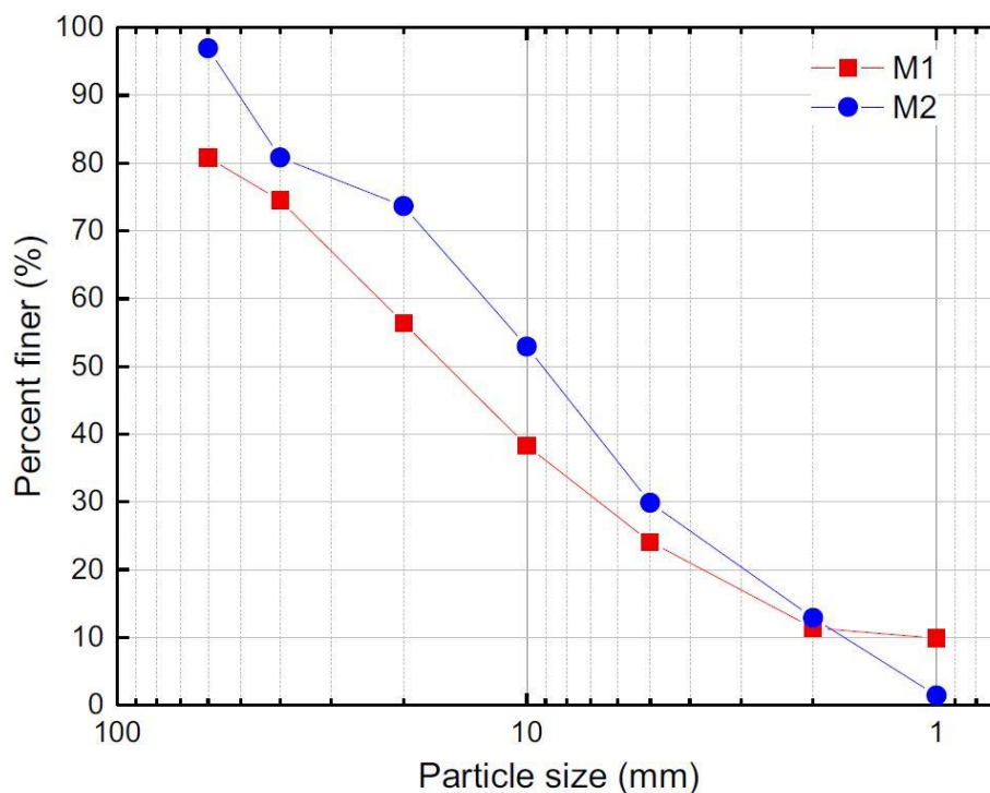
Slika 14. Granulometrijska analiza BMO uzoraka (Zhang i sur., 2020) (Prijevod: Os x – particle size (mm) – veličina čestica u mm; Os y – percent finer (%) – udio prolaza kroz sito)
