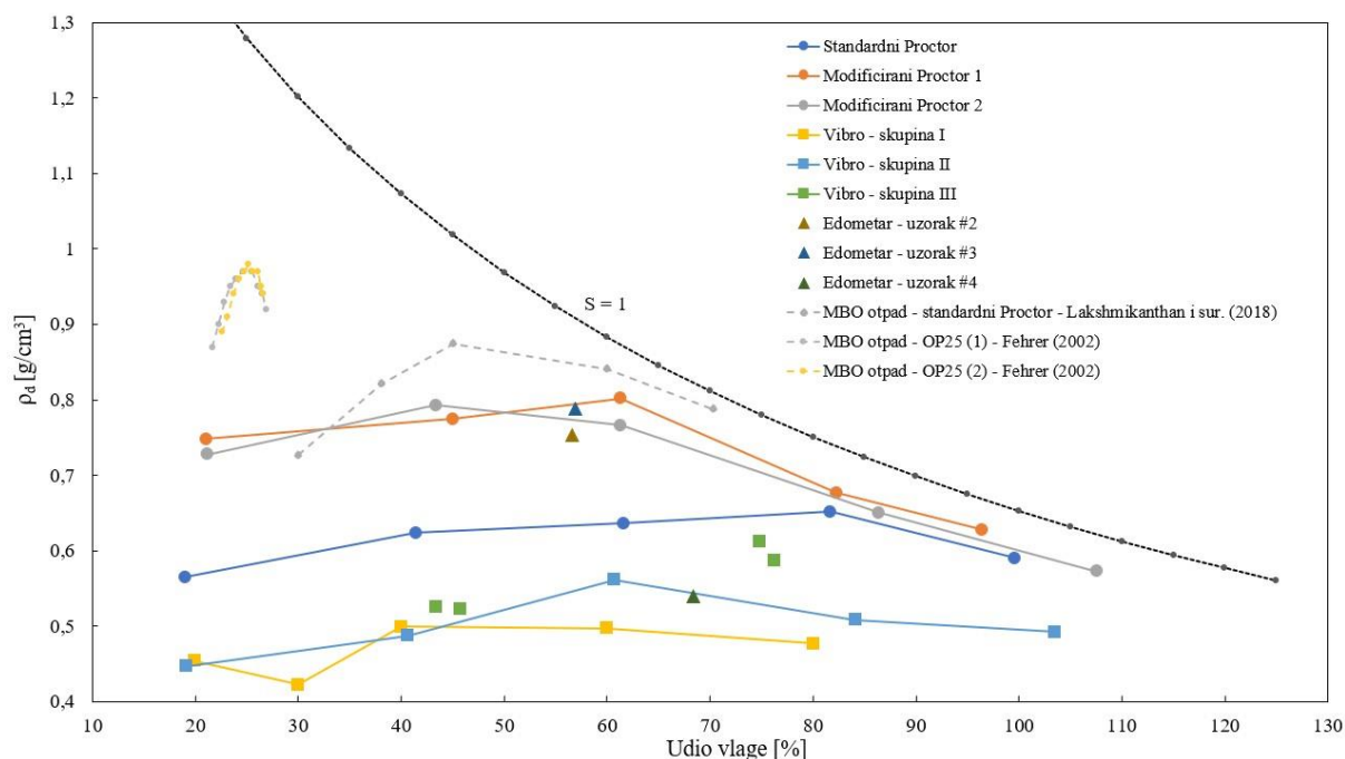
Slika 67. Proctorove krivulje izmjerene u ovom istraživanju u usporedbi s objavljenom literaturom
