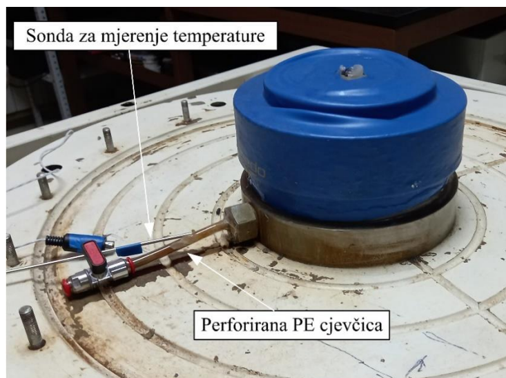
Slika 84. Edometarska ćelija: a) s geotekstilom na dnu, sondom za mjerenje temperature i perforiranom cjevčicom; b) s uzorkom, gumenom membranom, sondom za mjerenje temperature i perforiranom PE cjevčicom za mjerenje plinova i dodavanje vode
