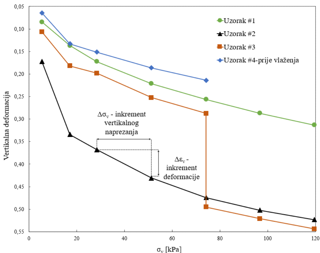
Slika 91. Odnos vertikalne deformacije i naprezanja uzoraka #1, #2, #3 i #4
