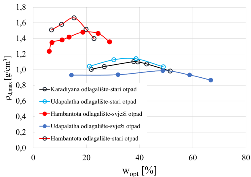
Slika 54. Krivulje zbijanja neobrađenog komunalnog čvrstog otpada (Iqbal i sur., 2022)
