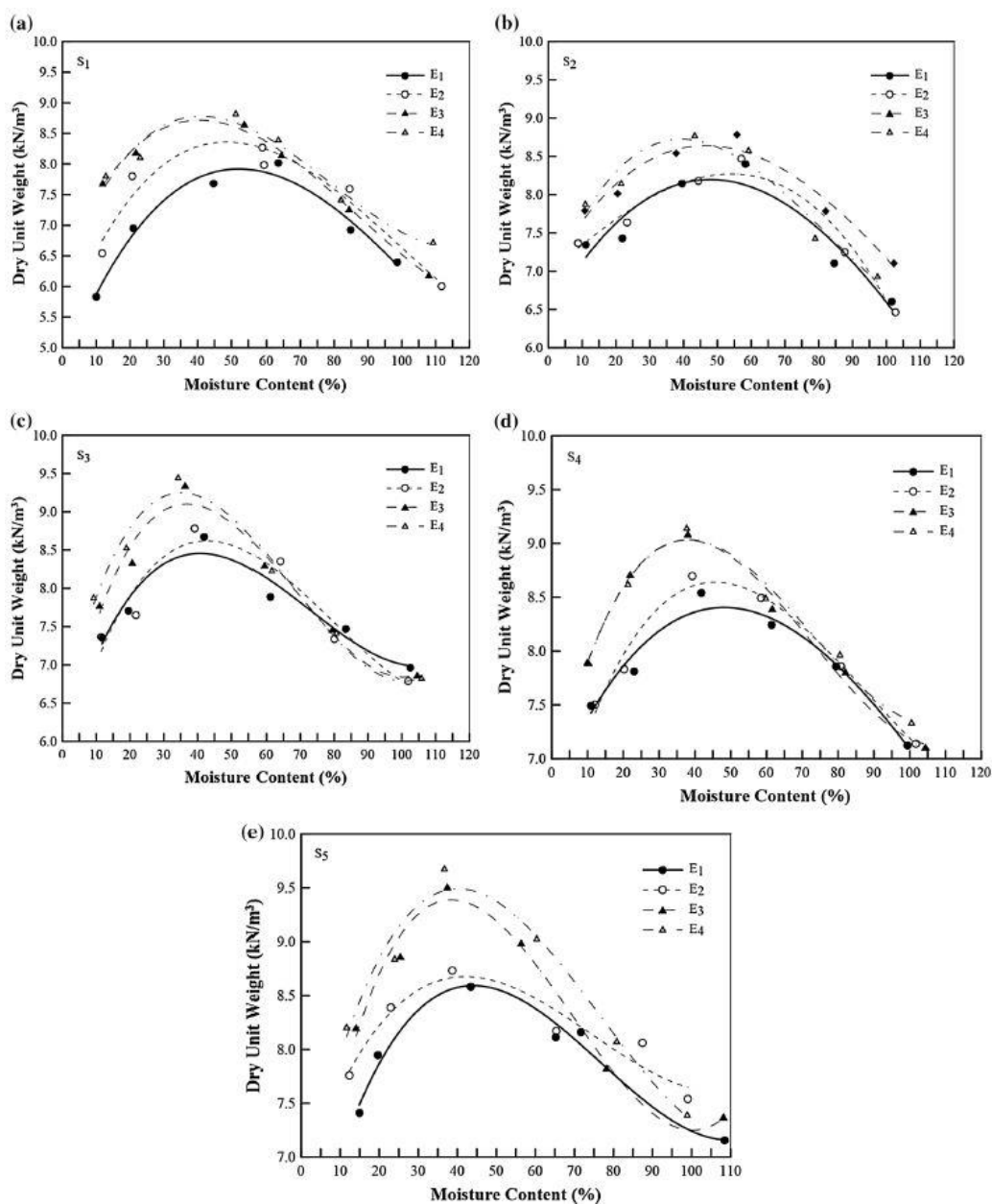
Slika 52. Krivulje zbijanja kod različitih energija zbijanja E_1 - E_4 : a) svježi otpad; b) otpad star 2 mjeseca; c) otpad star 5 godina; d) otpad star 10 godina; e) otpad star 15 godina (Endait i Patil, 2020) (Prijevod: Os x – moisture content (%) – udio vlage izražen kao postotak; Os y – dry unit weight ( \text{kN/m}^3 ) – suha zapreminska težina ( \text{kN/m}^3 ))
