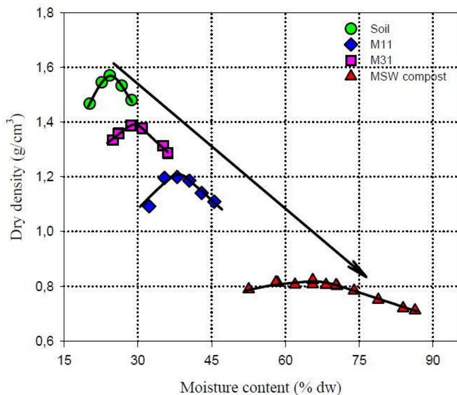
Slika 45. Krivulje zbijanja za četiri vrste materijala (Rose i sur., 2009) (Prijevod: Os x – moisture content (% dw) – udio vlage izražen kao postotak na suhu masu; Os y – dry density (g/cm³) – suha gustoća (g/cm³))
