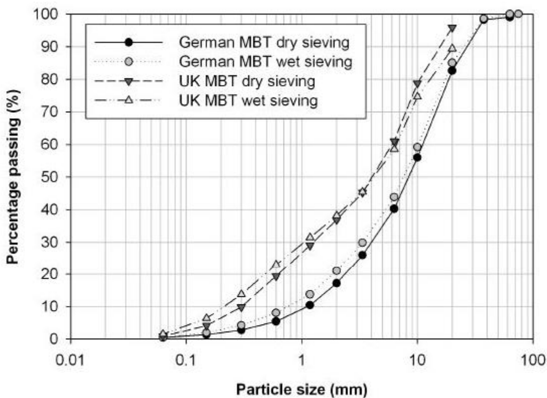
Slika 11. Granulometrijske krivulje MBO otpada iz Engleske i Njemačke za frakciju >5 mm, suho (dry) i vlažno (wet) prosijavanje (Velkushanova, 2011) (Prijevod: Os x – particle size (mm) – veličina čestica u mm; Os y – percentage passing (%) – udio prolaza kroz sito)
