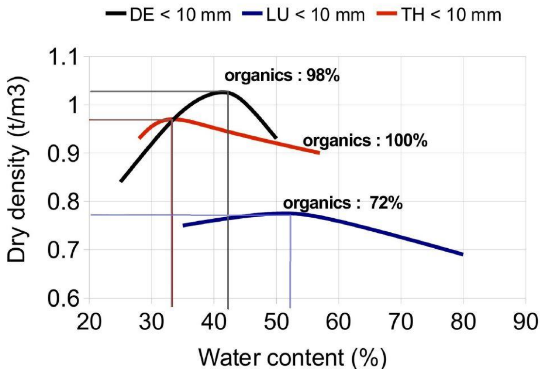
Slika 46. Rezultati zbijanja u standardnom Proctorovom pokusu neobrađenog otpada (Pimolthai, 2010) (Prijevod: Os x – water content (%) – udio vlage izražen kao postotak; Os y – dry density ( \text{t/m}^3 ) – suha gustoća ( \text{t/m}^3 ))
