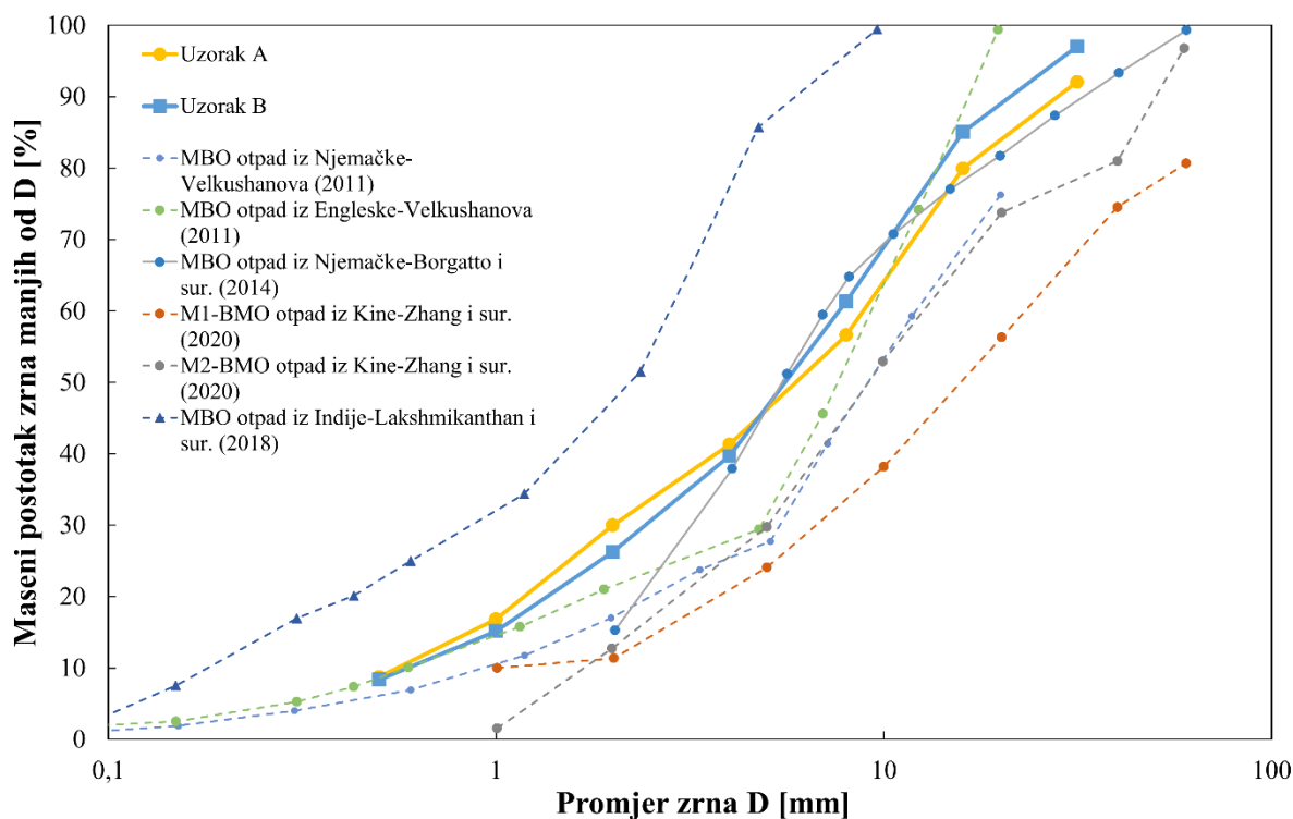
Slika 26. Granulometrijske krivulje vlastitih ispitivanja i ostalih istraživača
