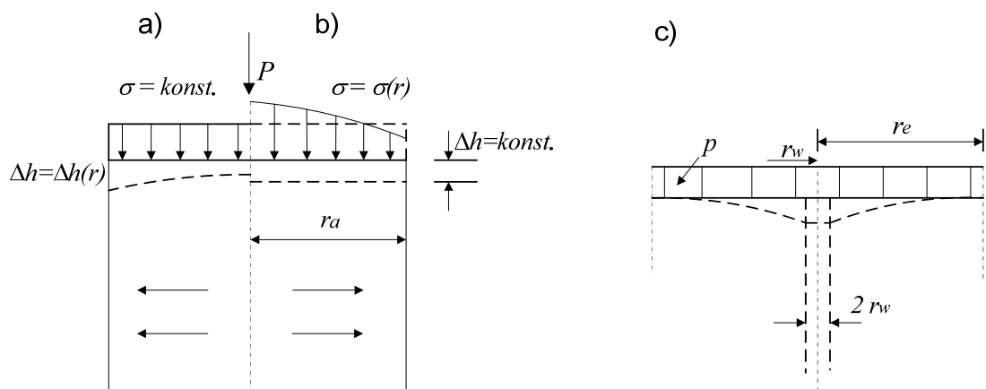
Slika 6. Ovisnost radialne konsolidacije oko dreva za različite načine opterećivanja površine: a) kontinuirano opterećenje, b) fleksibilno opterećenje, c) opterećenje preko krute plohe (iz Nonveiller, 1979).
