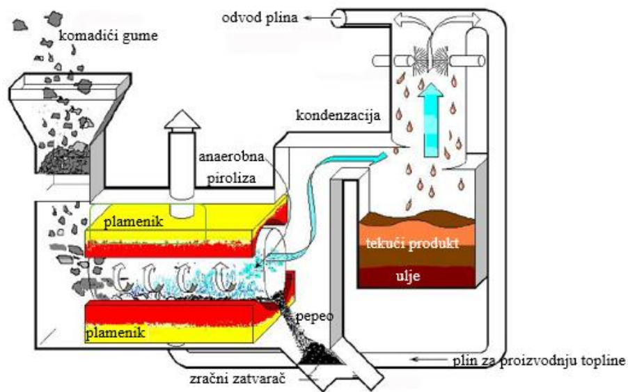
Slika 32. Postupak pirolize
