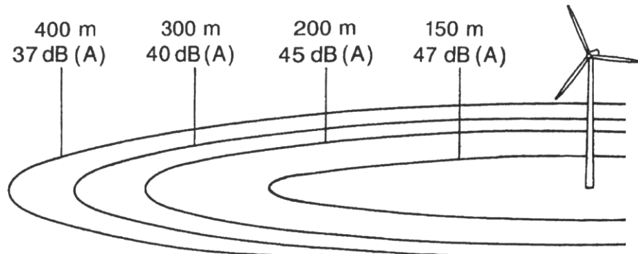
Slika 33. Intenzitet buke vjetroturbine na raznim udaljenostima od stupa vjetroturbine [35].
