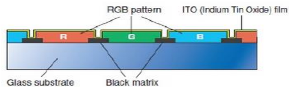
Slika 4 Filtri boja (5)
