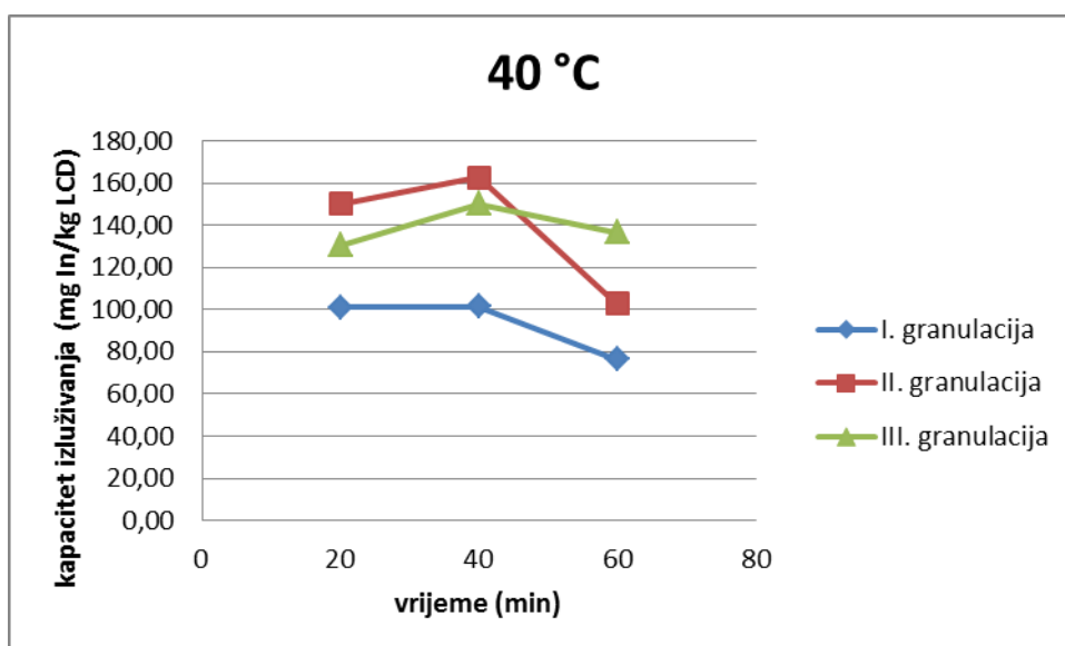
Slika 19 Kapacitet izluženog indija pri 40 °C
