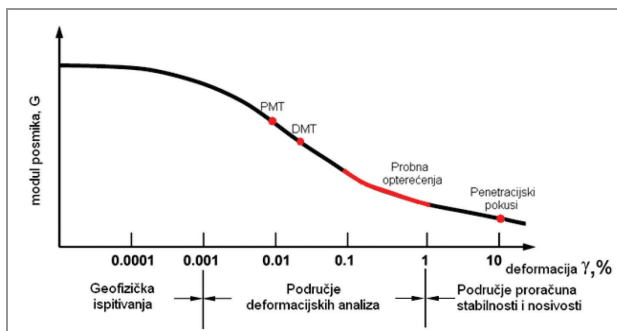
Slika 2. Raspodjela krutosti tla u ovisnosti o veličini deformacija i metodi ispitivanja (Luna, R., Jadi, H., 2000.)
