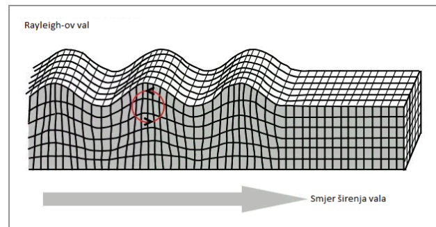
Slika 3. Širenje Rayleighevog vala
