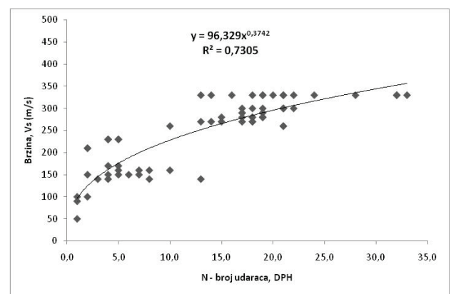
Slika 22. Korelacija v_s = f(N_{10H}) za istraživane krupnozrne šljunke
