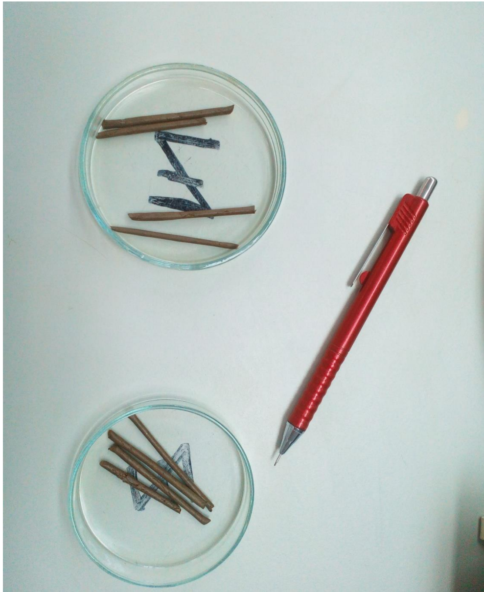
Slika 21. Valjčići za određivanje granice plastičnosti
