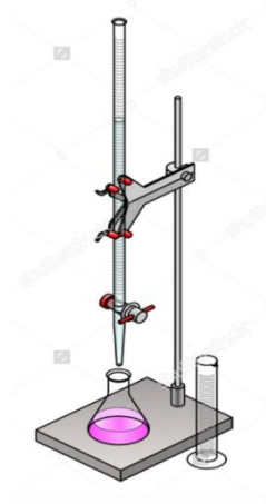
Slika 19. Aparatura za volumetrijsku titraciju
