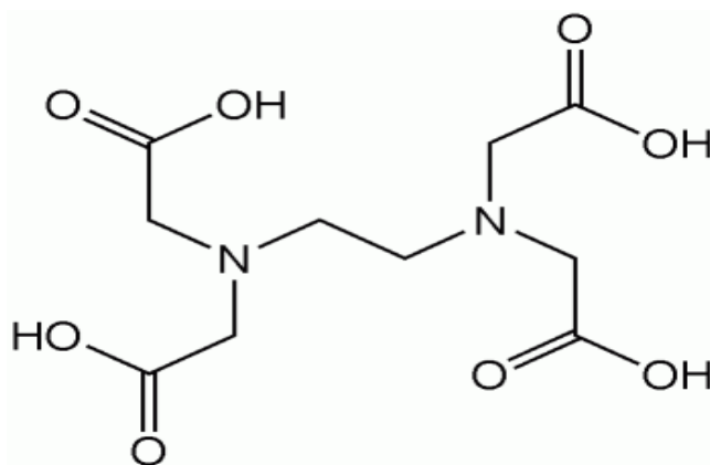
Slika 20. Etilendiamin-tetraoctena kiselina
