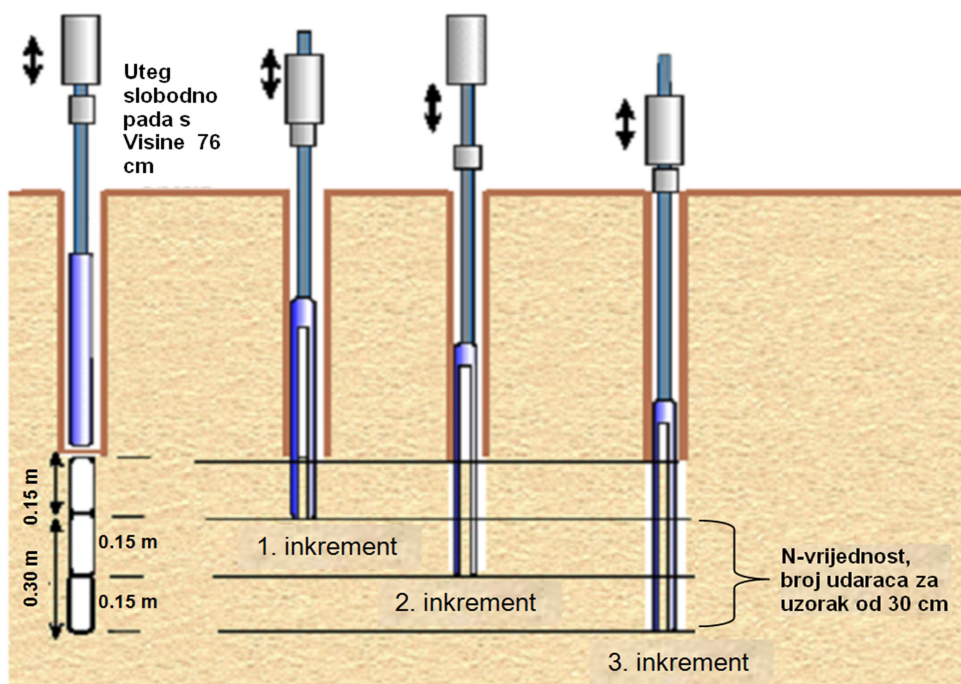
Slika 6. Postupak ispitivanja standardnim penetracijskim pokusom (Roje-Bonacci,2012)
