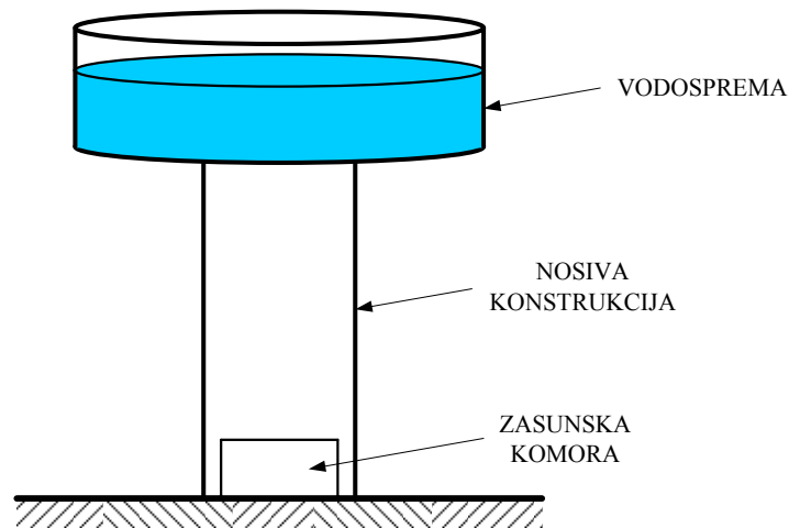
Slika 5. Vodotoranj (Margeta, 2011)
