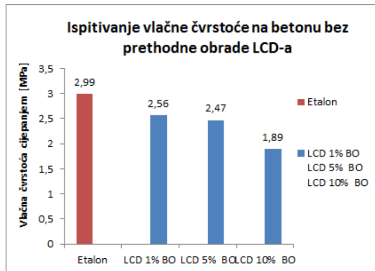
Slika 23. Ispitivanje vlačne čvrstoće za beton bez prethodne obrade LCD – a
