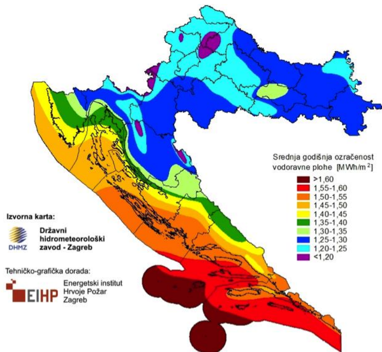
Slika 2. a) Solarni potencijal za proizvodnju električne energije na području Republike Hrvatske; b) srednja godišnja ozračenost horizontalne ravnine i solarni potencijal [2,4]
