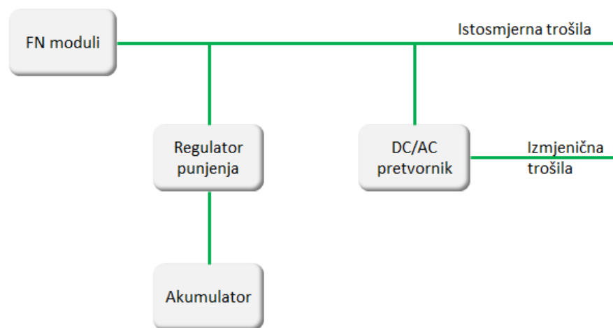
Slika 3. Samostalni FN sustav za istosmjerna i izmjenična trošila [8]
