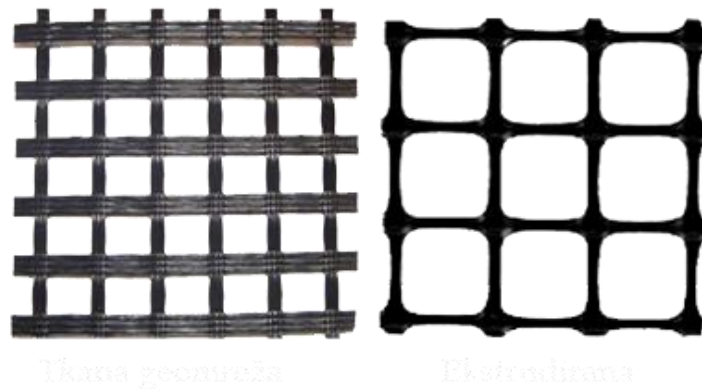
Slika 9. Geomreža [12]
