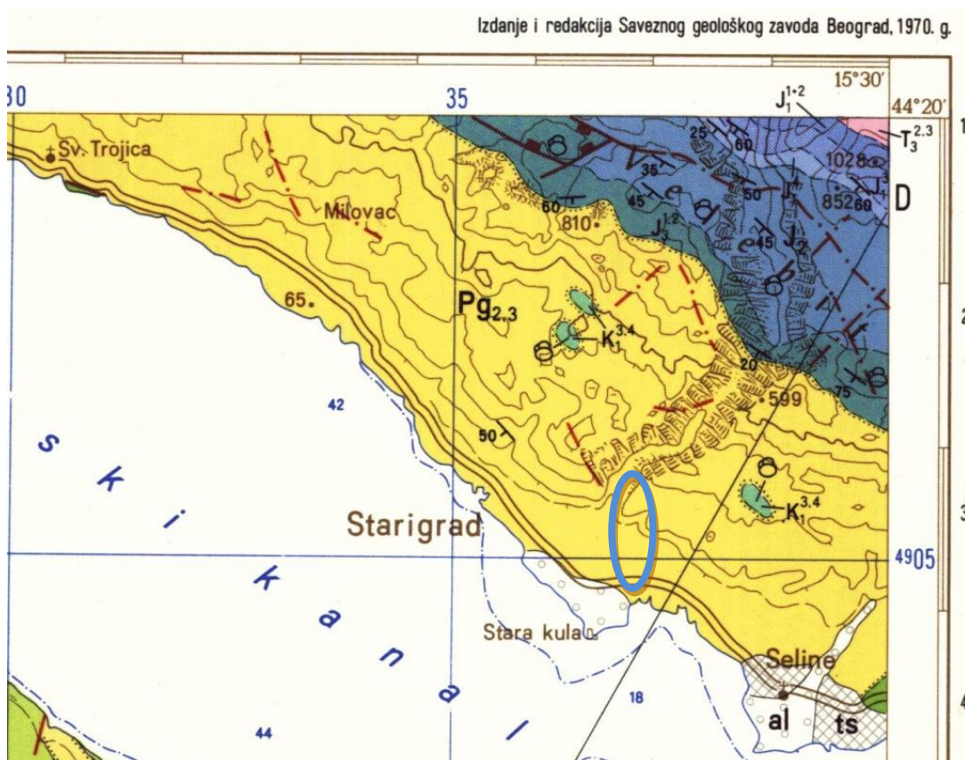
Slika 1. Položaj trase ceste na osnovnoj geološkoj karti.(Coley, 2014).
